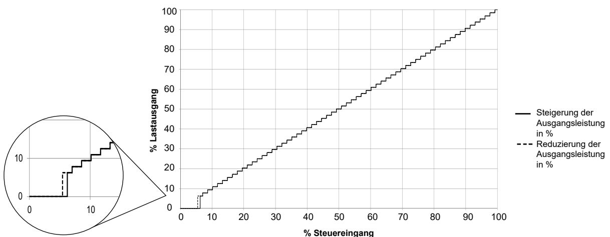
16-fachpuls-Schaltmodus: RGC...C16
