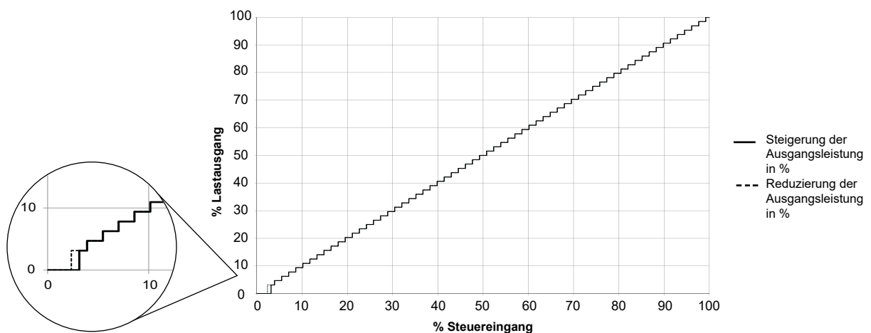
Vierfachpuls-Schaltmodus: RGC...C4
