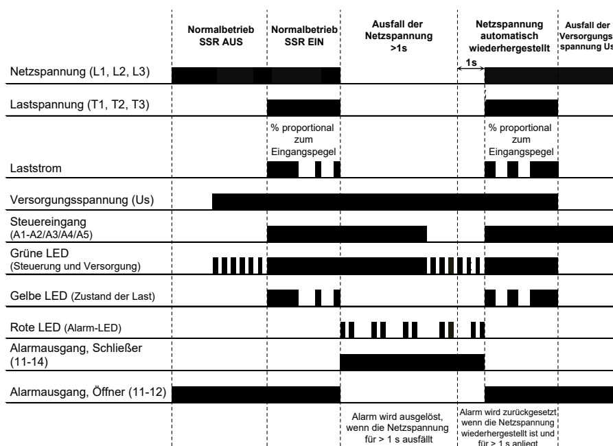
Betriebsdiagramm 3:
