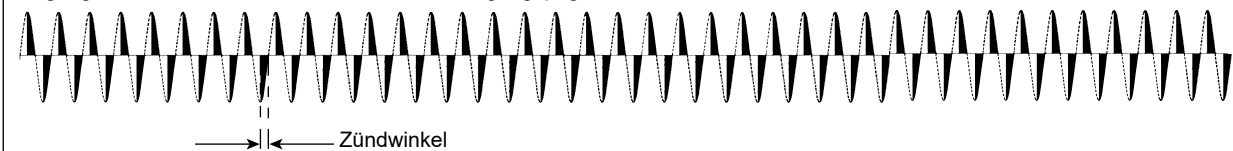
Ausgang im Phasenanschnitt-Schaltmodus bei Eingangspegel 50 %:
