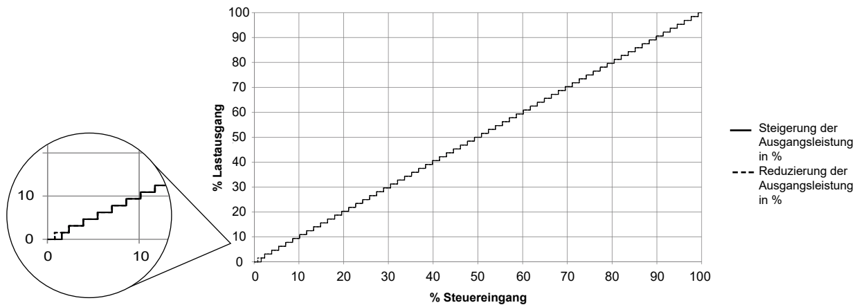
Einzelpuls-Schaltmodus: RGC...C1
