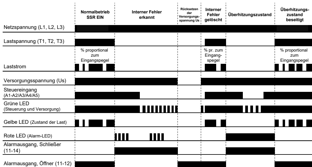
Betriebsdiagramm 3:
