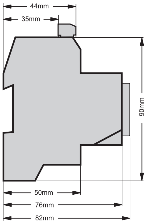
Seitenansicht
