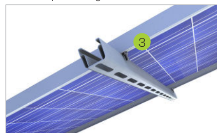
Modulabrutschsicherung an der Rahmenbohrung für Modulhochkantmontage
