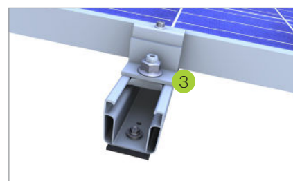
Modulabrutschsicherung an der Rahmenbohrung für Modulquermontage
