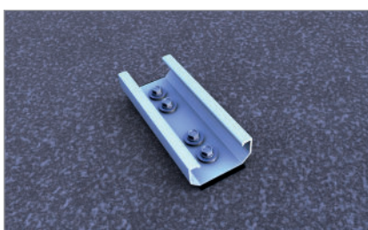
Kurzprofil C24 mit vier Dichtschrauben für hohe Windlast
