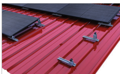
Variante mit quer aufgeständerten Modulen
