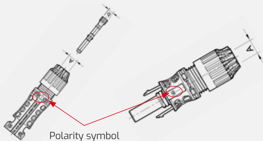
Abb. 7: Kennzeichnung der Polarität auf den MC4-Evo2 Steckverbindern
