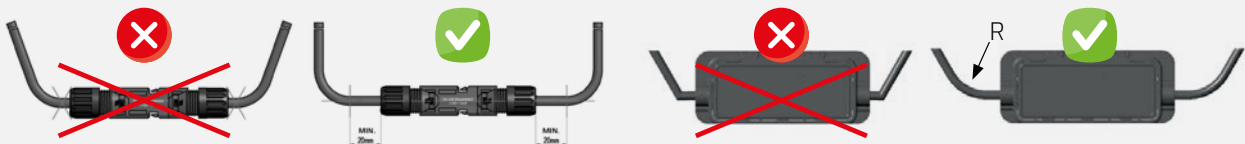
Abb. 5: zulässiger Biegeradius der Solarkabel
