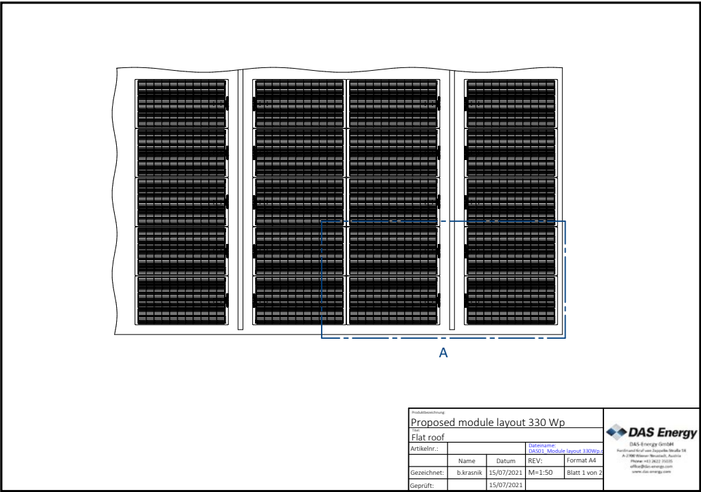
Abb. 1: Beispiel eines typischen Belegungsplanes für Flachdächer (Modultyp 11x6 FJB) – Überblicksansicht
