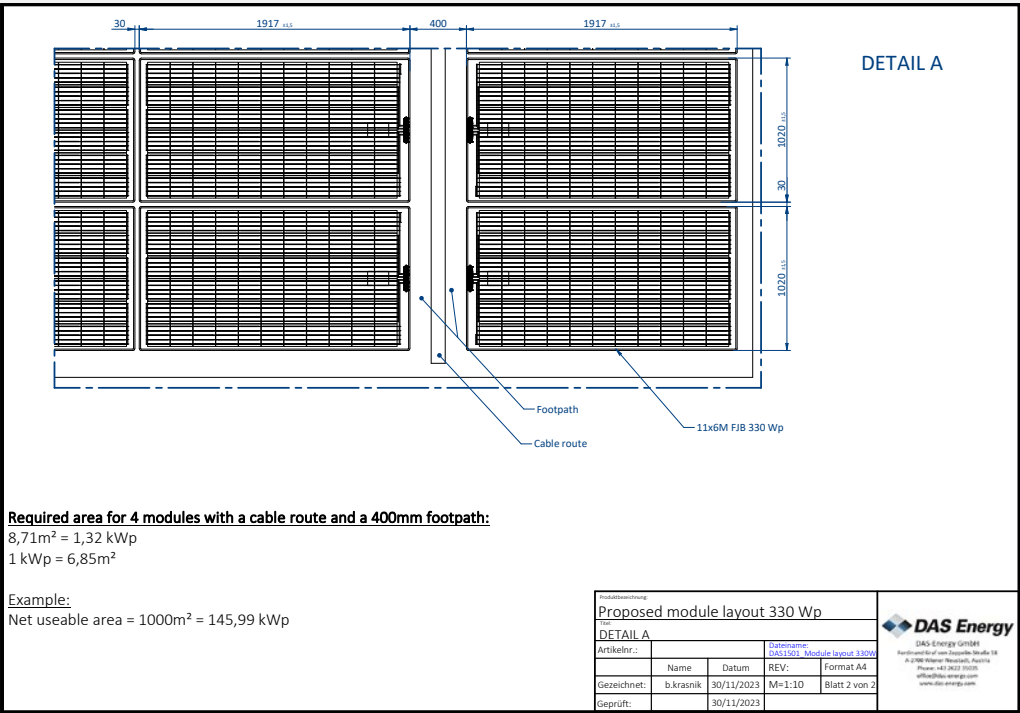
Abb. 2: Beispiel eines typischen Belegungsplanes für Flachdächer mit 50 mm Kabel-tasse (Modultyp 11x6 FJB) – Detailsicht
