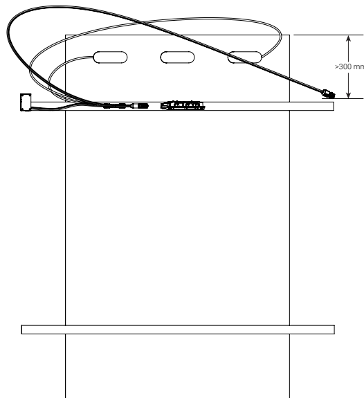
Abbildung 4: Vertikale Montage
