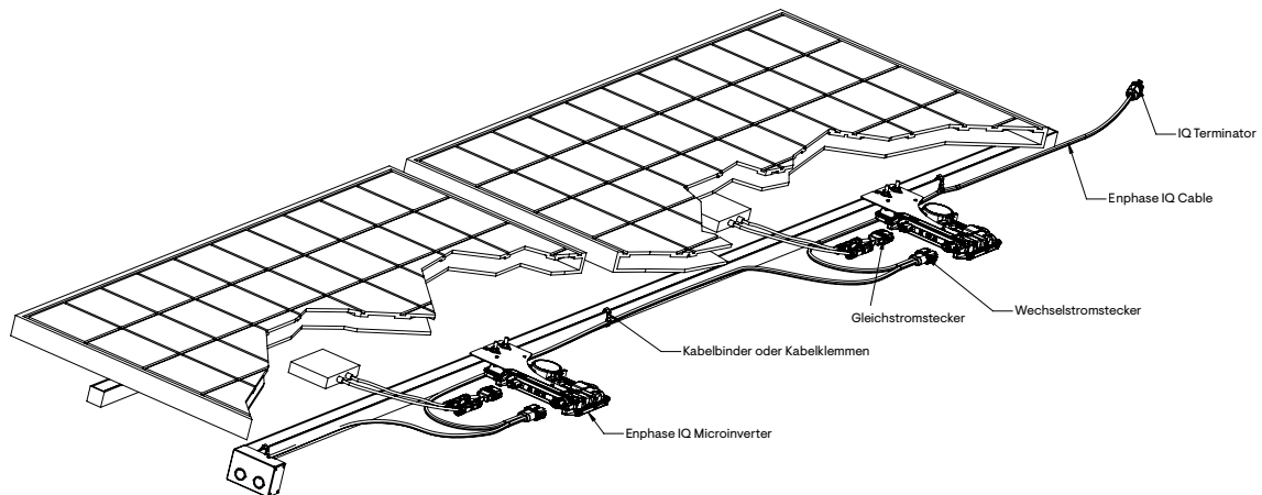
Abbildung 1: Horizontale Montage
