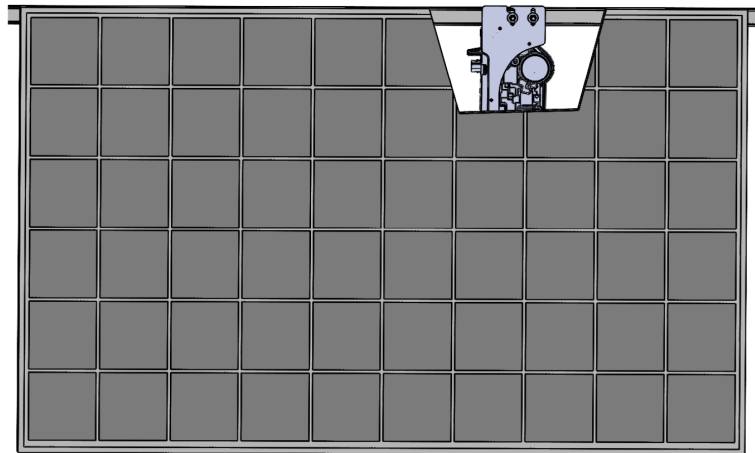
Abbildung 3: Horizontale Montage
