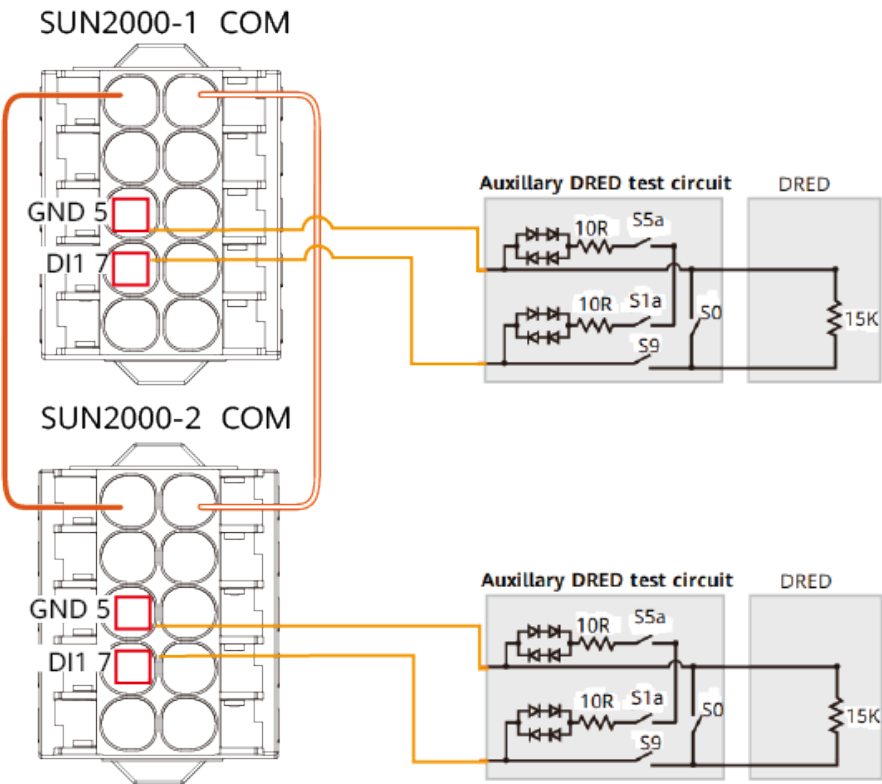
Abbildung 7-4 Schaltplan für die DRM-Funktion
