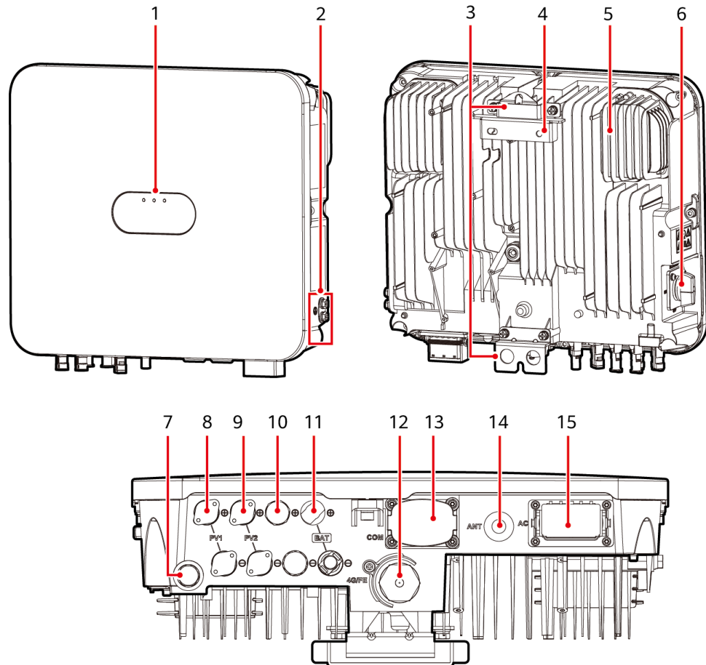
Abbildung 2-6 Erscheinungsbild
