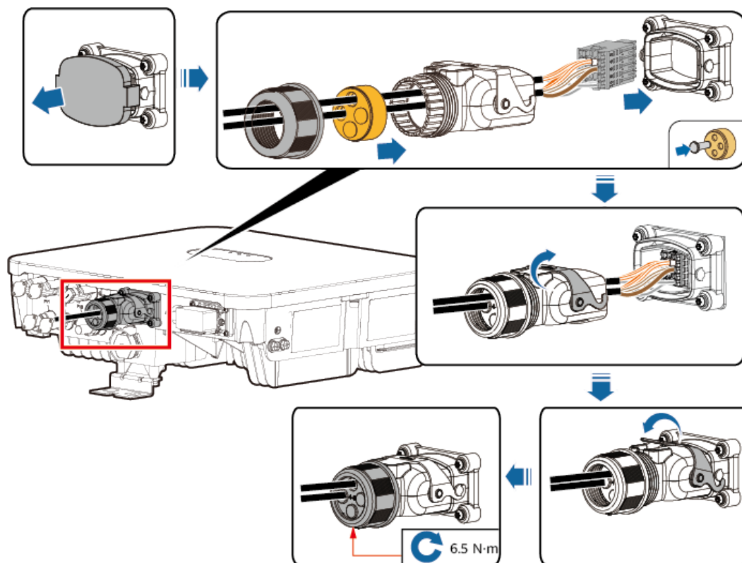
Abbildung 5-31 Sichern des Signalkabelsteckverbinders
