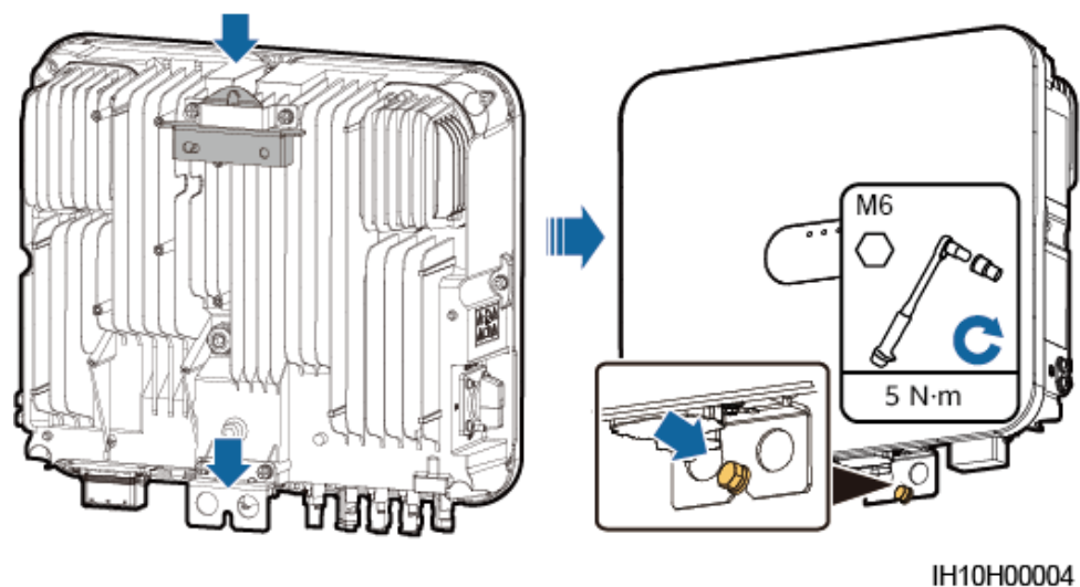
Abbildung 4-14 Festziehen der Schrauben
