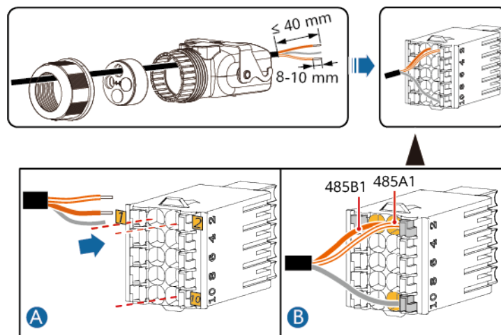
Abbildung 5-21 Anschließen der Kabel (Verbinden mit der SmartAssistant)
