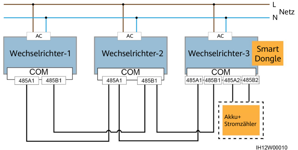
Abbildung 5-14 Smart Dongle-Vernetzung (die Komponenten in gestrichelten Kästen sind optional)
