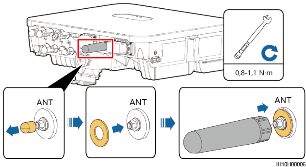
Abbildung 5-38 Montieren einer WLAN-Antenne
