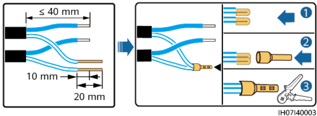
Abbildung 5-16 Crimpen zweier Signalkabel
