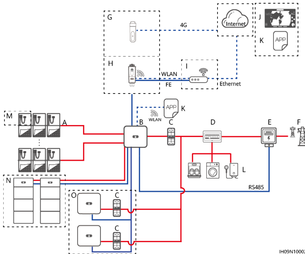
Abbildung 2-3 Smart Dongle-Vernetzung (die Komponente im gestrichelten Kasten ist optional)
