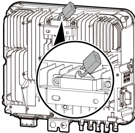
Abbildung 4-10 Montieren eines Diebstahlschutz-Schlusses
