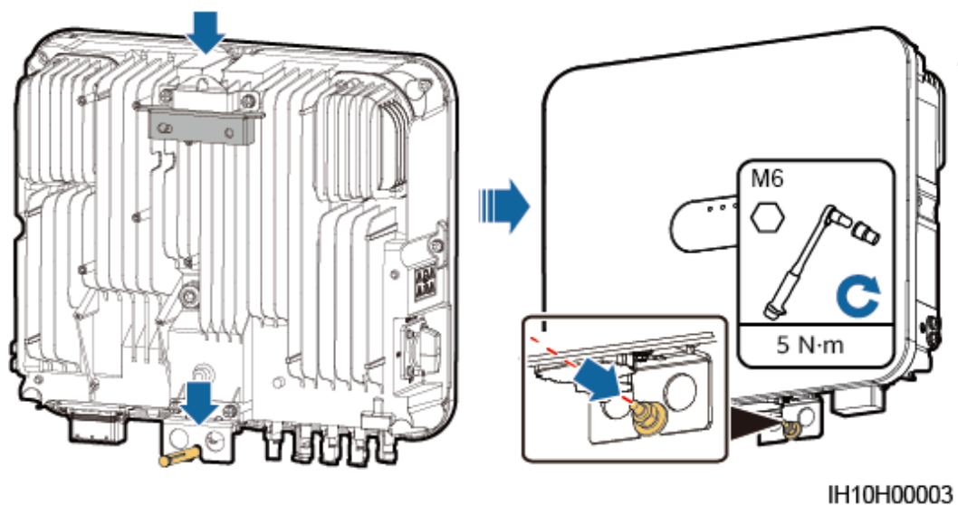
Abbildung 4-9 Anziehen der Muttern
