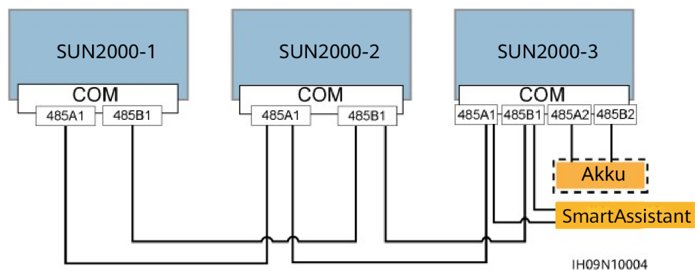
Abbildung 5-15 SmartAssistant-Vernetzung (die Komponente im gestrichelten Kasten ist optional)
