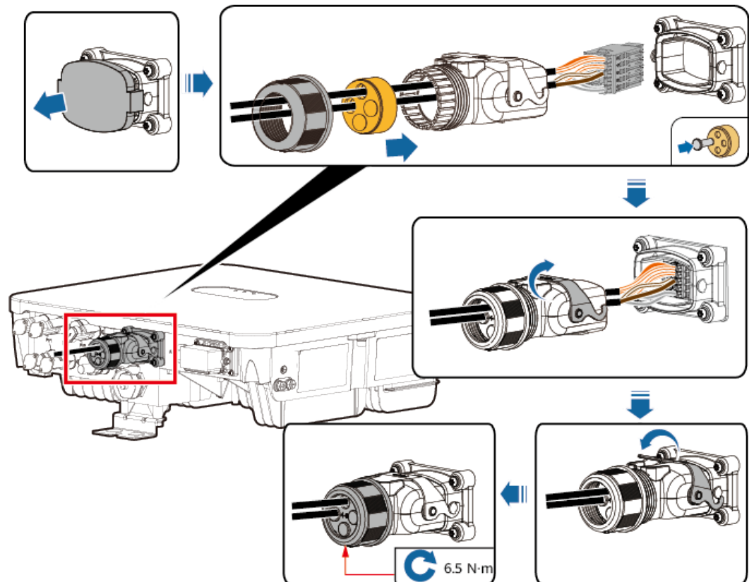
Abbildung 5-23 Sichern des Signalkabelsteckverbinders
