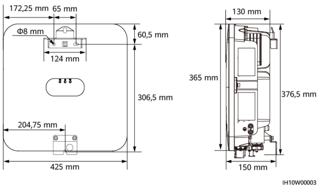
Abbildung 4-1 Abmessungen der Montagehalterung
