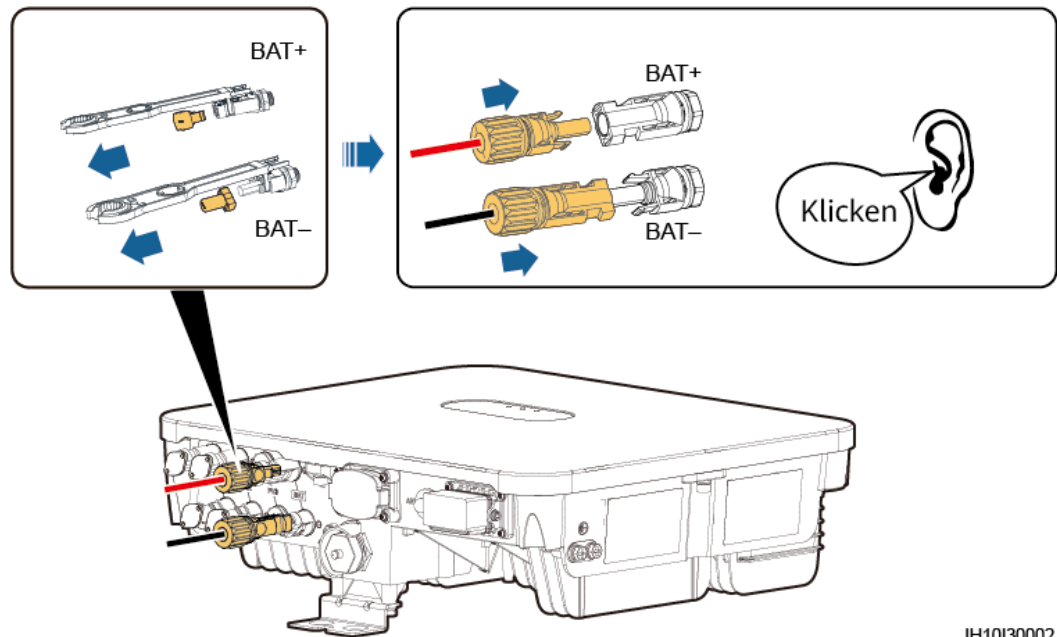
Abbildung 5-12 Anschließen der Batteriekabel
