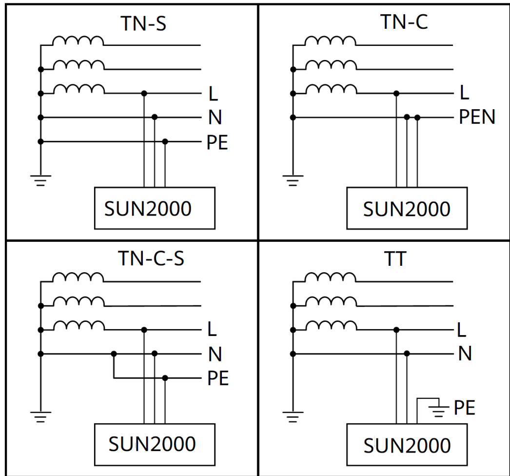
Abbildung 2-5 Erdungssysteme
