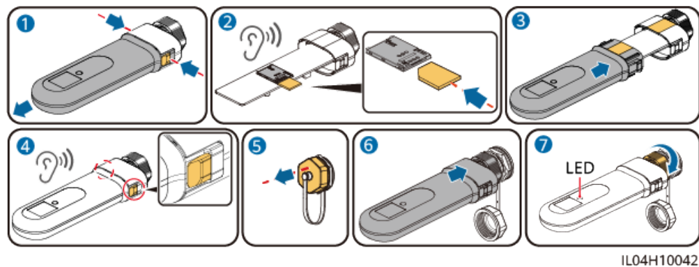
Abbildung 5-36 Installieren von 4G Smart Dongle (SDongleB-06)
