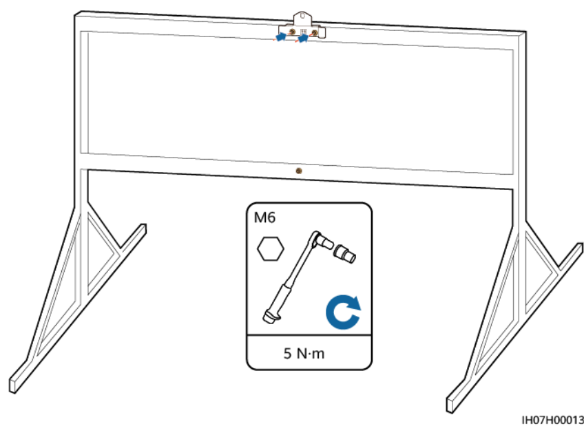
Abbildung 4-13 Sichern der Montagehalterung
