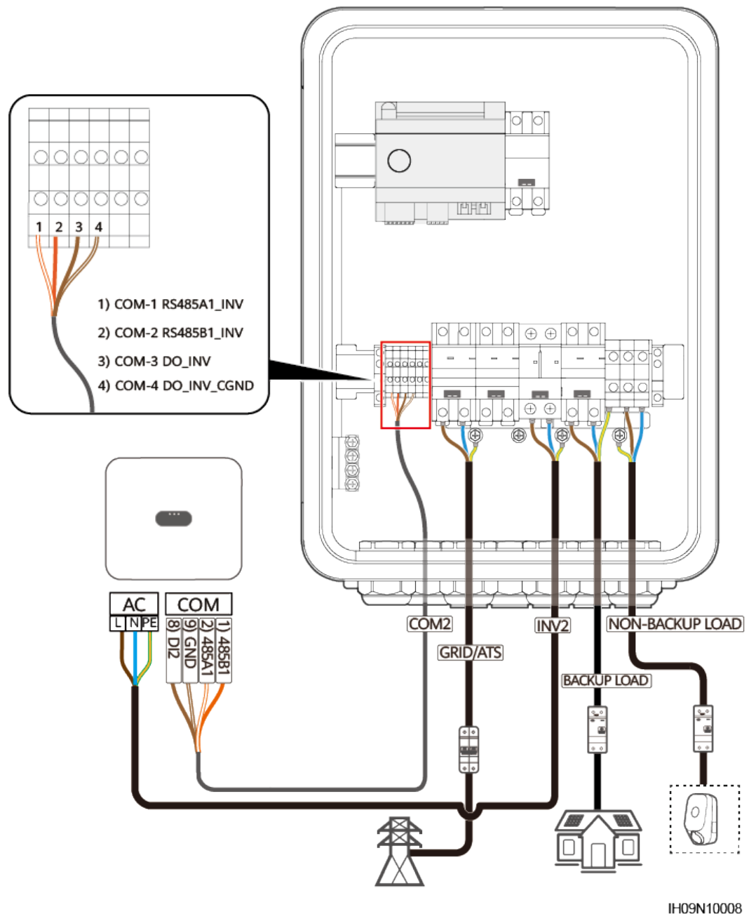
Abbildung 5-24 Anschließen von Kabeln an SmartGuard
