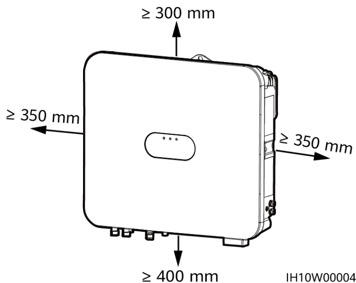
Abbildung 4-2 Abstände
