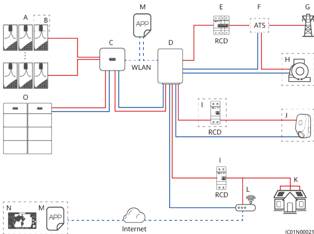
Abbildung 2-4 SmartGuard-Vernetzung (die Komponenten in gestrichelten Kästchen sind optional)
