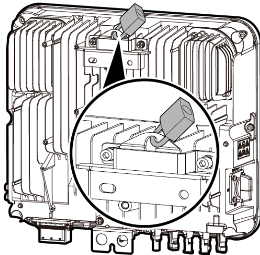
Abbildung 4-15 Montieren eines Diebstahlschutz-Schlusses
