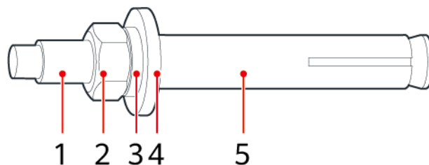
Abbildung 4-7 Aufbau einer Dehnschraube
