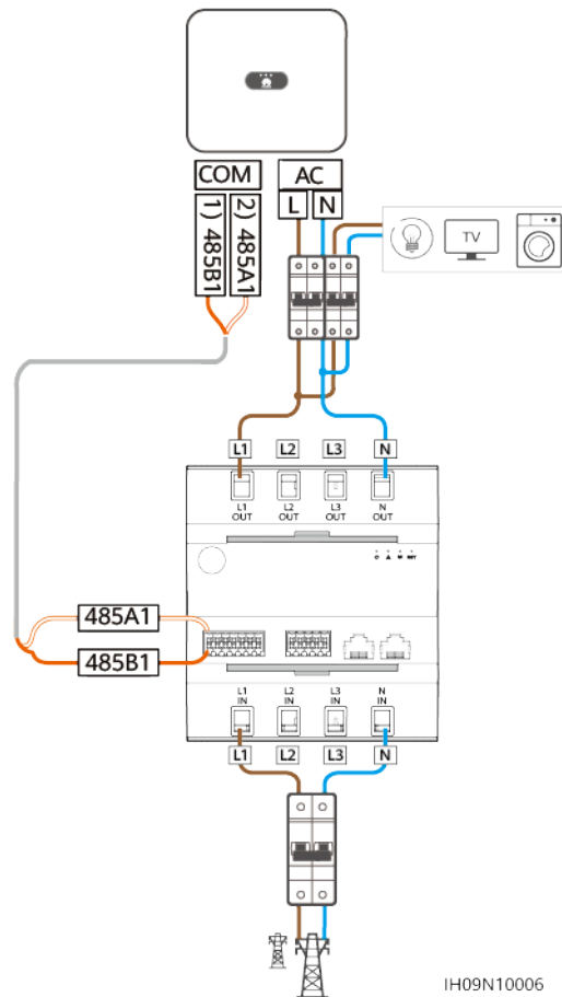
Abbildung 5-20 Anschließen von Kabeln an die SmartAssistant
