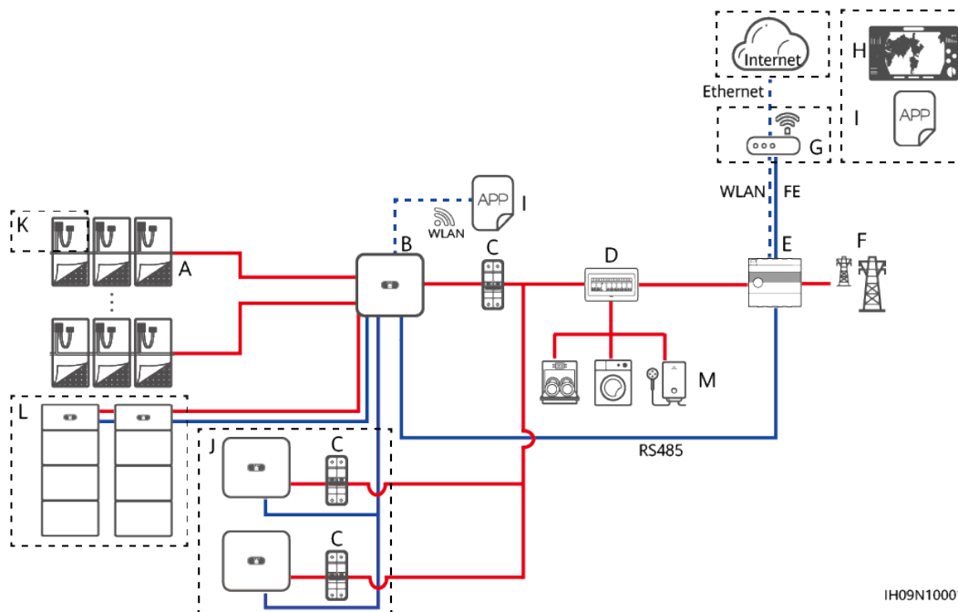
Abbildung 2-2 SmartAssistant-Vernetzung (die Komponenten im gestrichelten Kasten sind optional)
