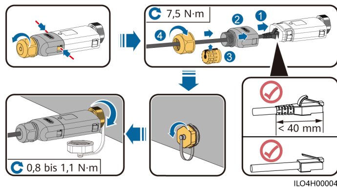
Abbildung 5-34 Installieren von WLAN-FE-Smart Dongle (FE-Kommunikation)
