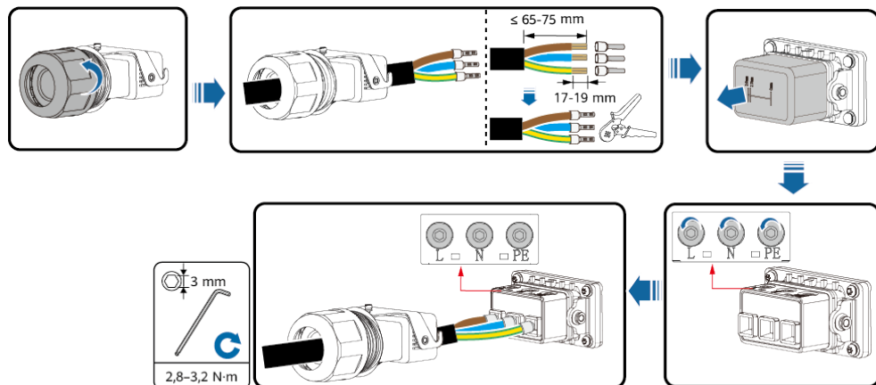
Abbildung 5-4 Anschließen des AC-Stromkabels
