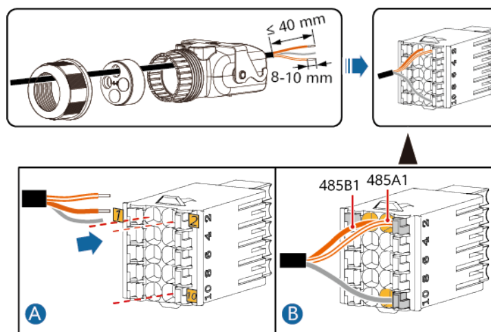
Abbildung 5-18 Installieren des Kabels
