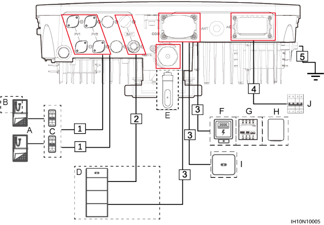
Abbildung 5-1 Kabelanschlüsse des Wechselrichters (die Komponenten im gestrichelten Kasten sind optional)
