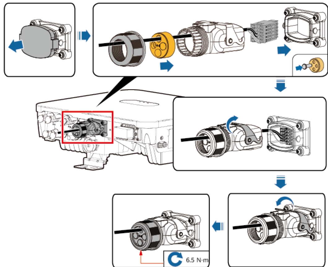
Abbildung 5-33 Sichern des Signalkabelsteckverbinders
