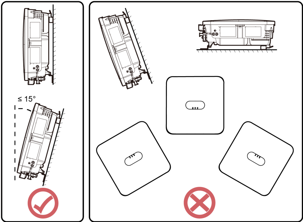
Abbildung 4-5 Montagewinkel
