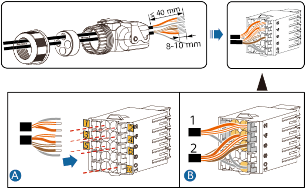
Abbildung 5-22 Anschließen der Kabel (Verbinden mit der SmartAssistant und Akku)
