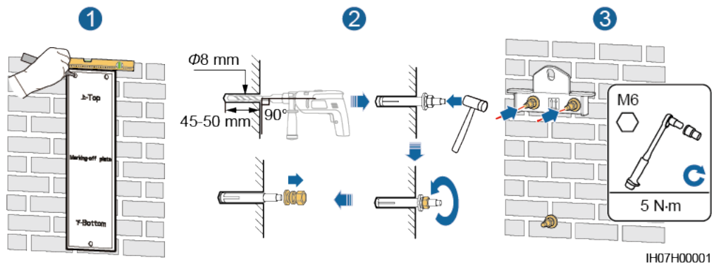
Abbildung 4-8 Einsetzen der Dehnschrauben
