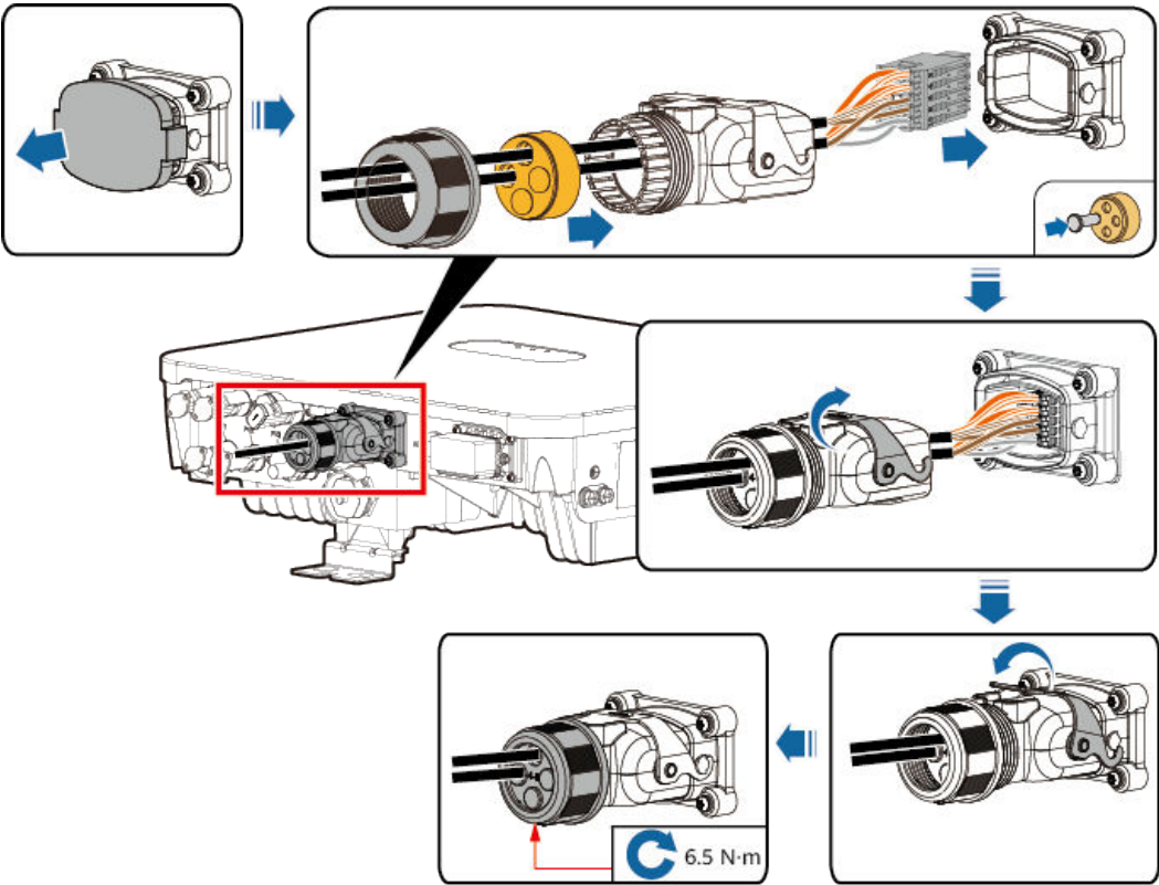
Abbildung 5-27 Sichern des Signalkabelsteckverbinders
