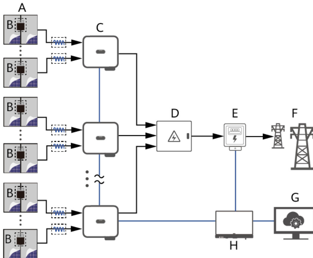
Abbildung 2-2 RS485-Vernetzung (SmartLogger)
