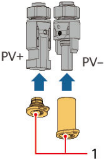
Abbildung 5-22 Verschlussstopfen
