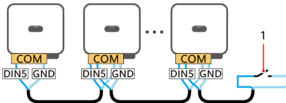
Abbildung 5-45 Anschließen von kaskadierten Wechselrichtern an den NS-Schutzschalter
