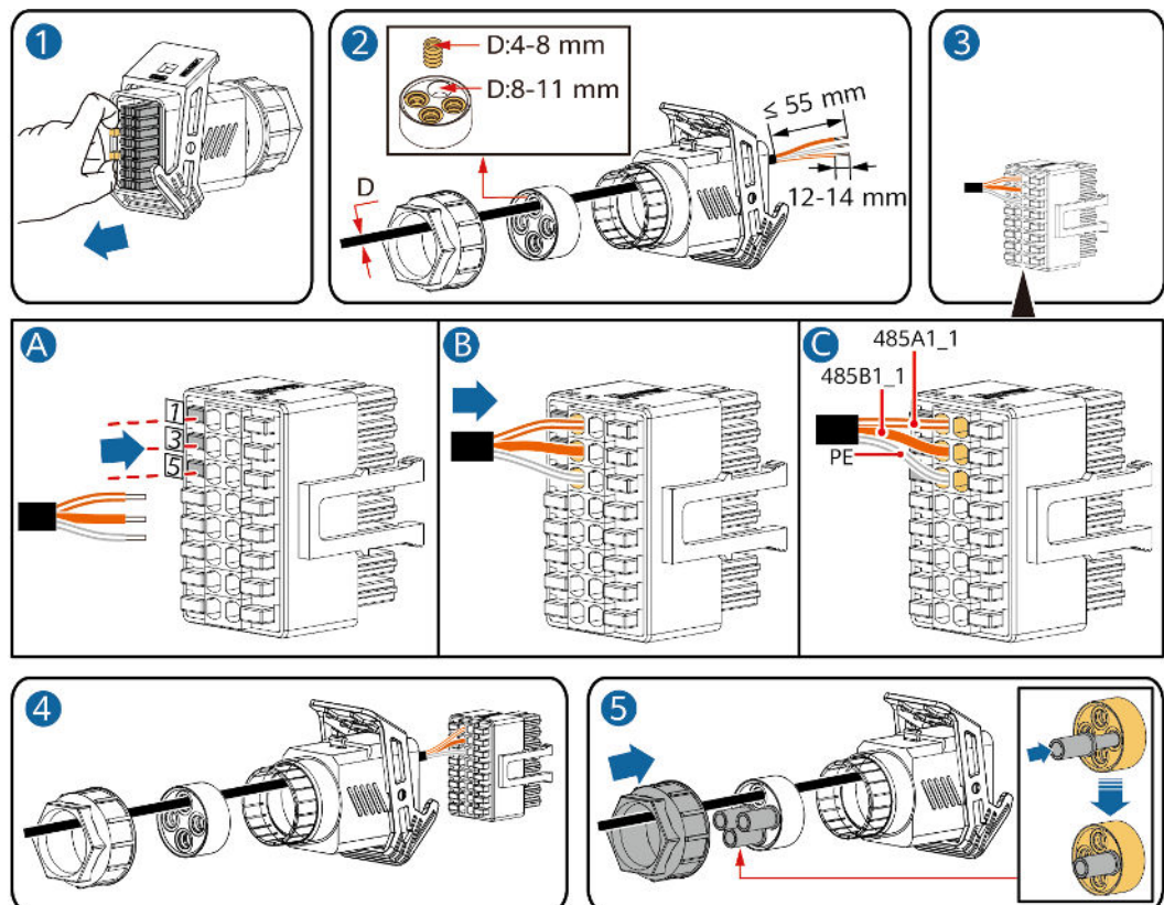
Abbildung 5-34 Kabelmontage
