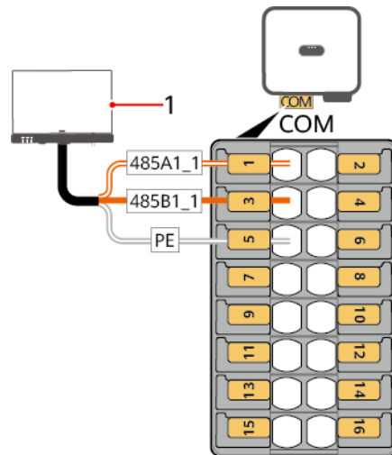
Abbildung 5-33 Kabelverbindung
