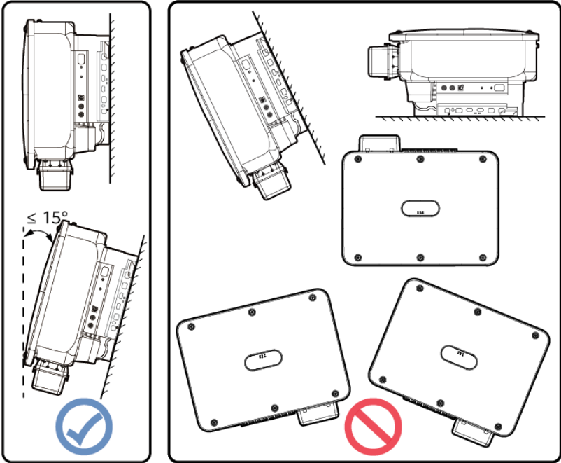
Abbildung 4-9 Installationswinkel
