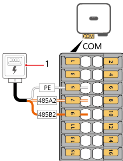
Abbildung 5-36 Kabelverbindung
