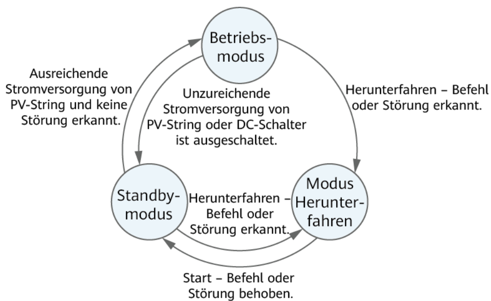
Abbildung 2-9 Arbeitsmodi
