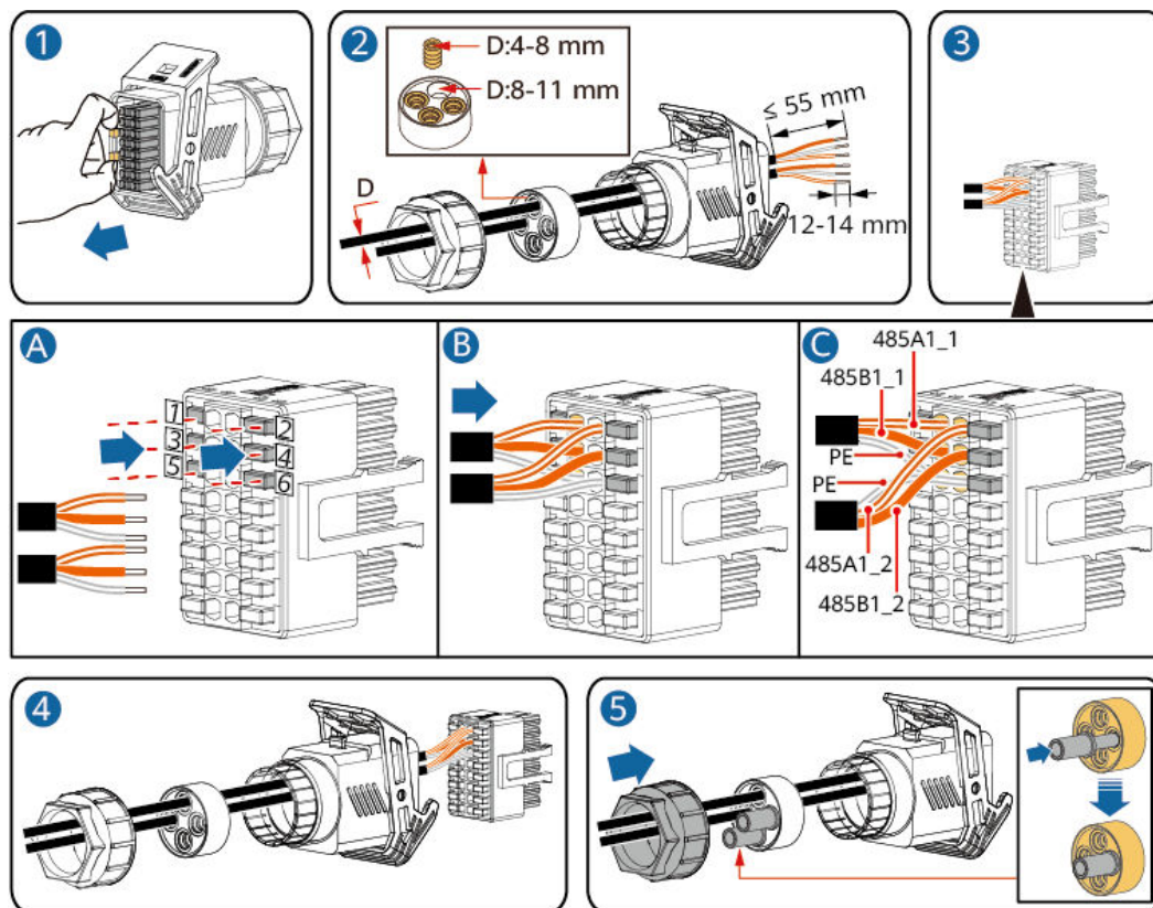
Abbildung 5-31 Kabelmontage
