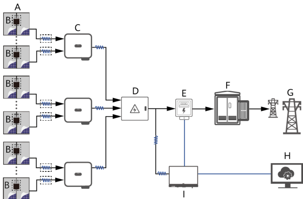
Abbildung 2-4 MBUS-Vernetzung (SmartLogger)
