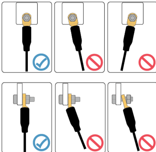
Abbildung 5-11 Verdrahtungsanforderungen
