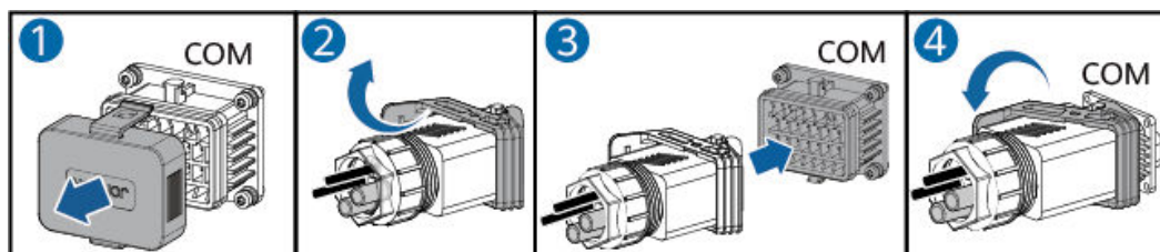
Abbildung 5-32 Sichern des Signalkabelsteckverbinders
