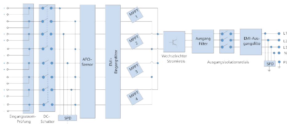
Abbildung 2-8 Schematisches Diagramm
