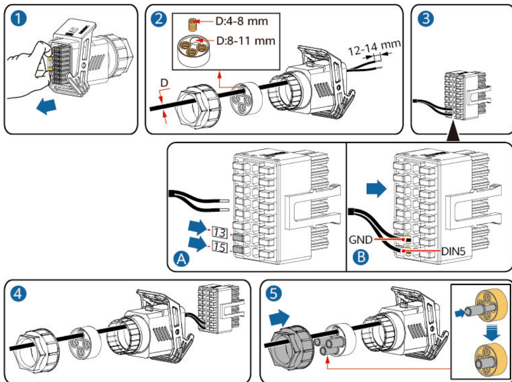
Abbildung 5-43 Kabelmontage
