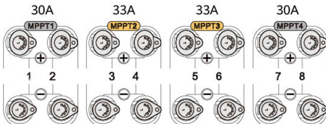
Abbildung 5-12 DC-Eingangsklemmen
