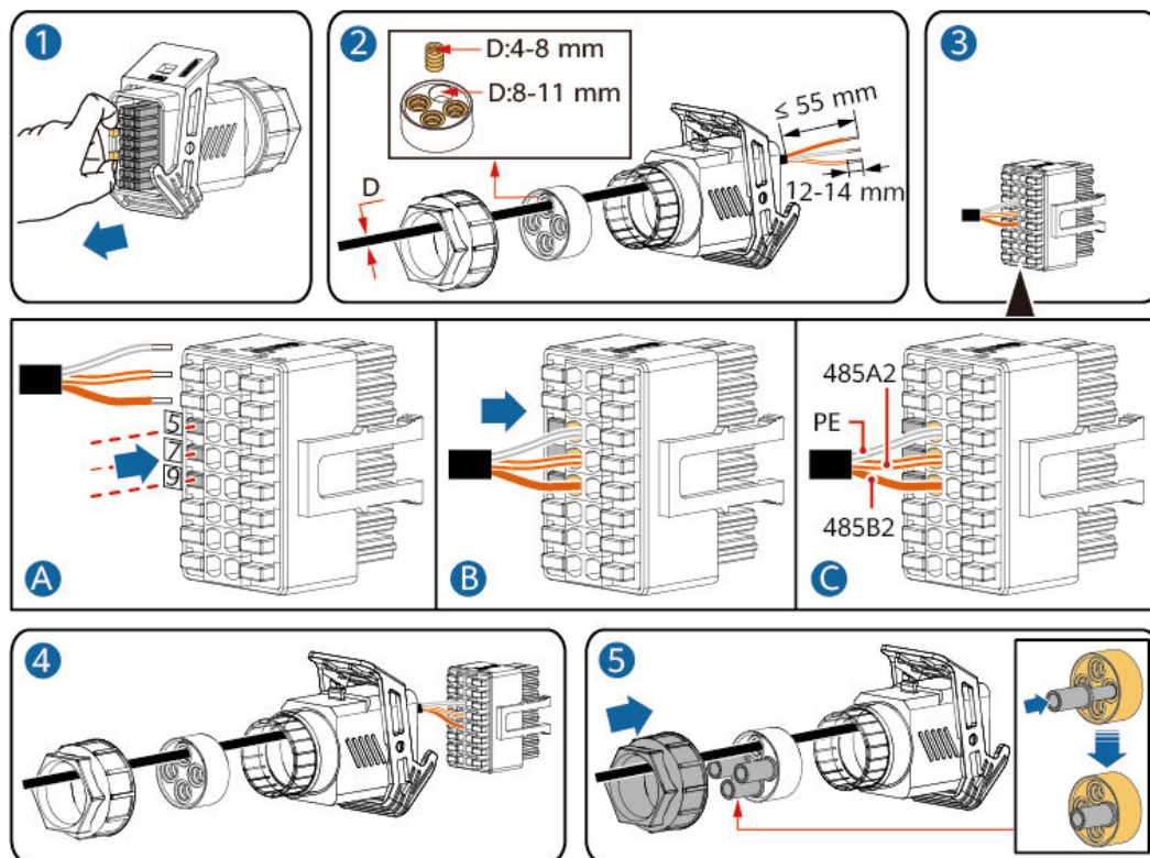
Abbildung 5-37 Kabelmontage
