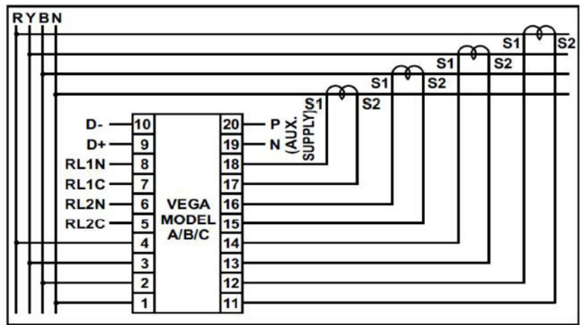
Abb.: Pin-Belegung
