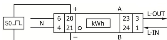
Abb.: Pin-Belegung
