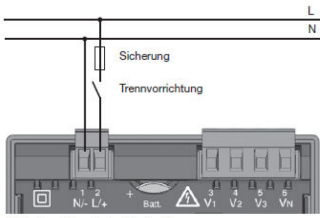
Abb.: Anschlussbeispiel „Versorgungsspannung“
