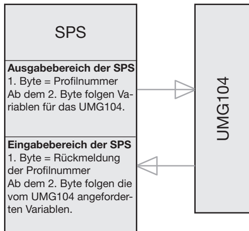
Abb.54.1 Blockschaltbild für den Datenaustausch zwischen SPS und UMG104.
