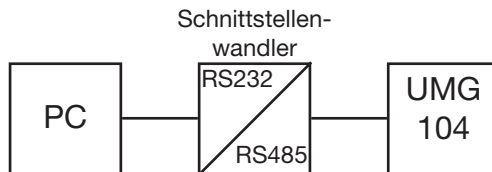
Abb.13.2 Anschluss eines UMG104 an einen PC über einen Schnittstellenwandler.
