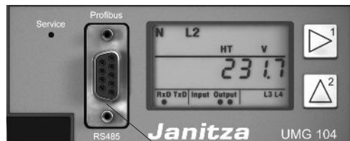
Abb.36.1 UMG104 mit Profibusschnittstelle.
