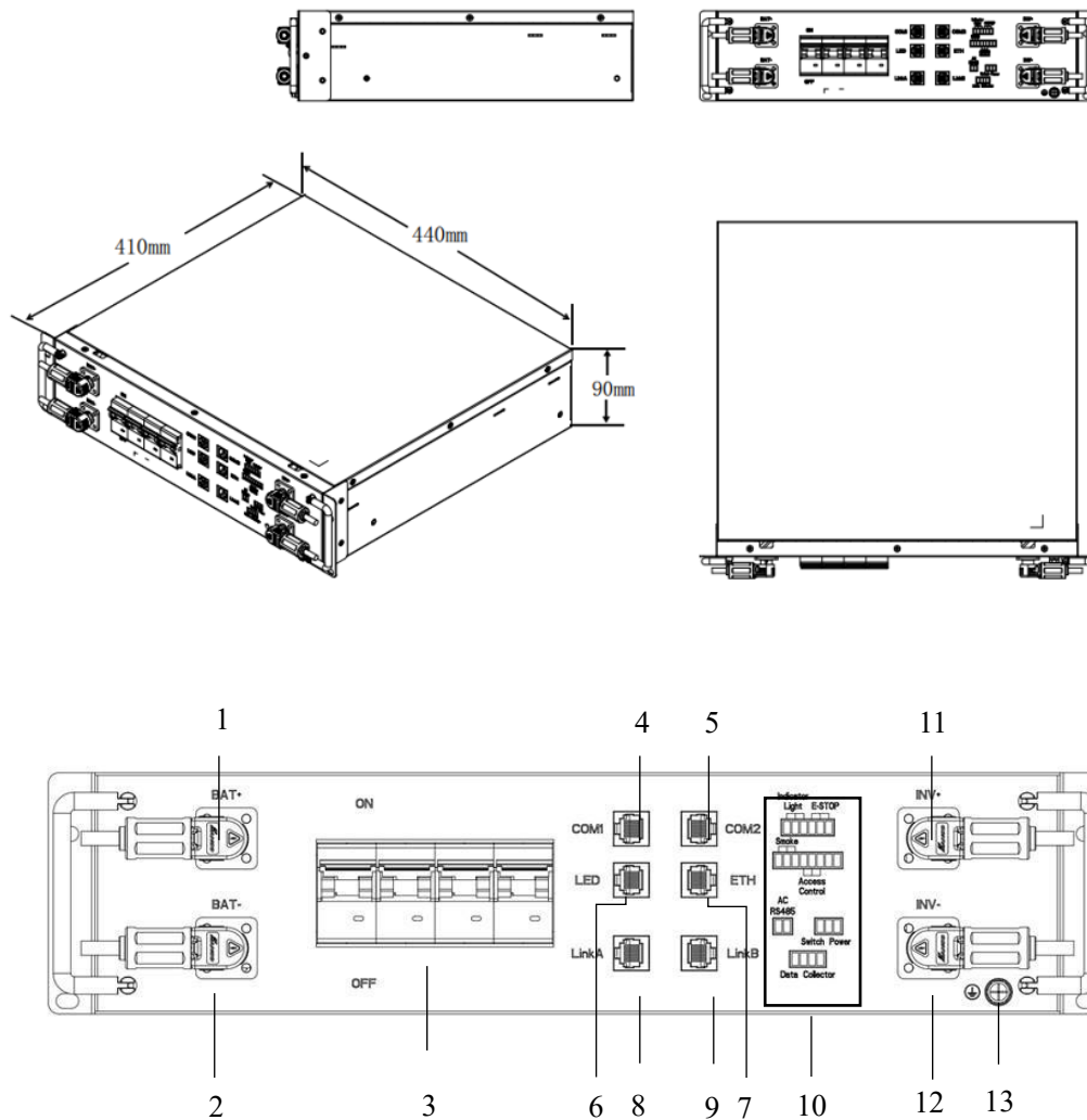
Abbildung 2.2.3 Steuerbox
