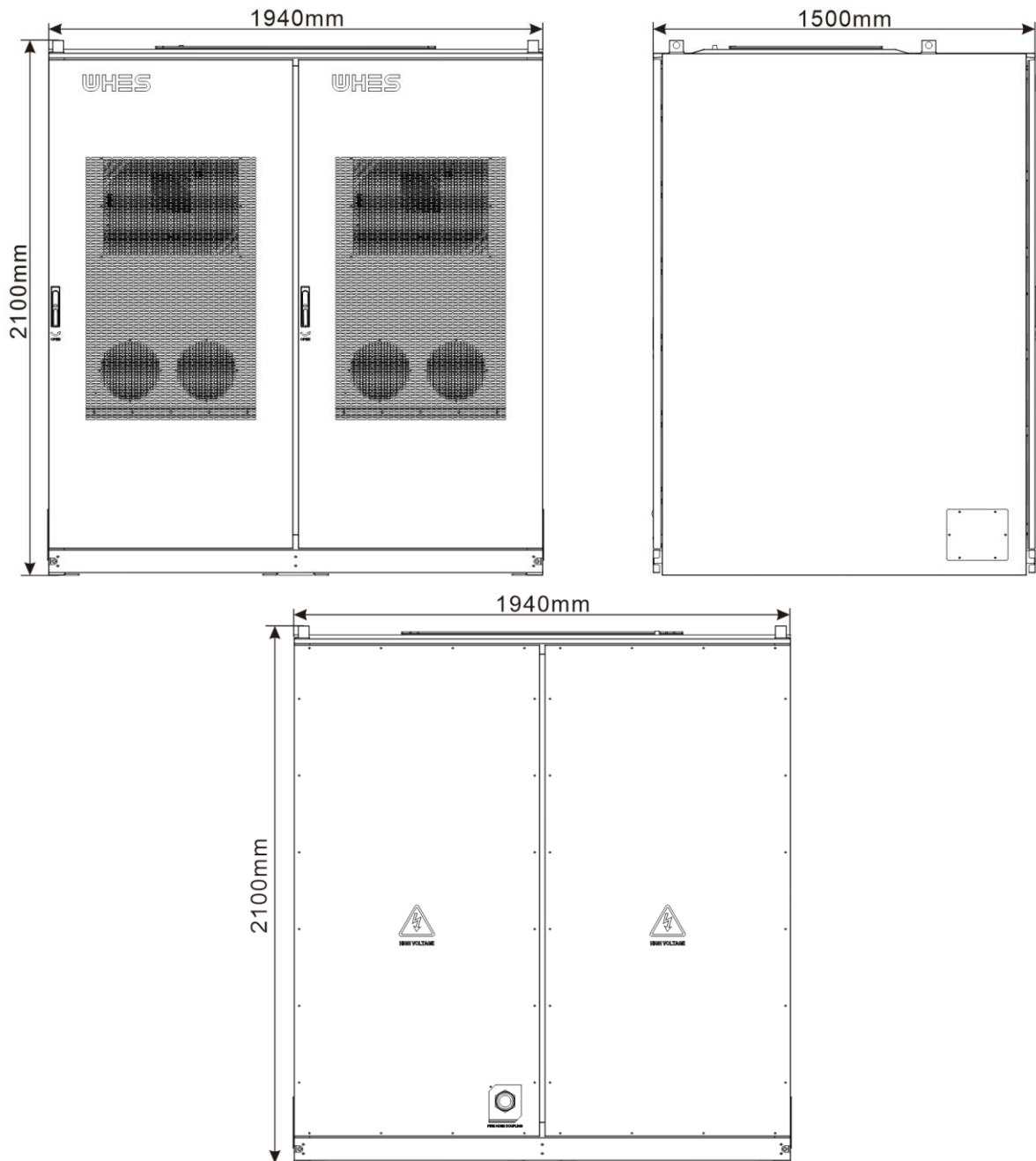
■ Abbildung 2-1 Aussehen und Abmessungen
