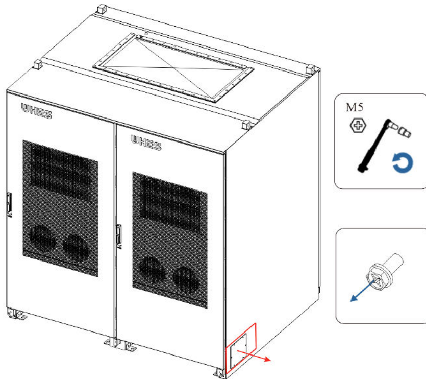
Abbildung 4-3 Zerlegen Sie die Verdrahtungsdichtungsplatte
