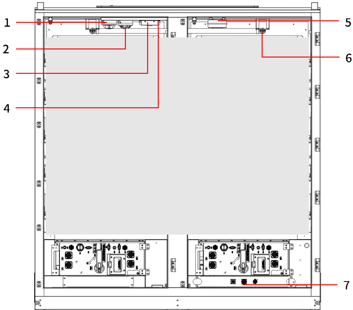
Abbildung 2-4 Batterieschrank – Innenraum – 2
