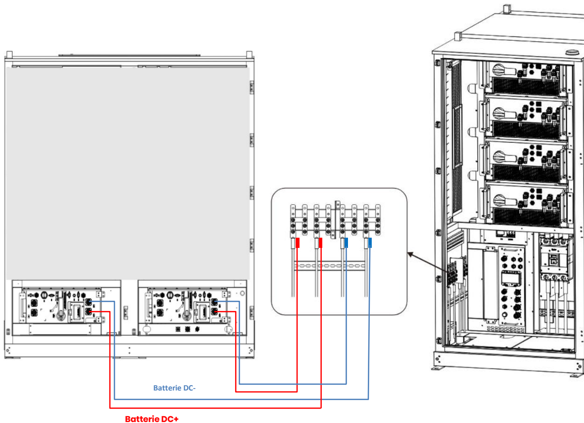
Abbildung 4-16 Installieren Sie die AC/DC-Kabel
