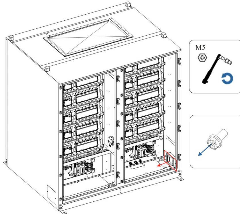
Abbildung 4-13 Zerlegen Sie die Spulendruckplatten
