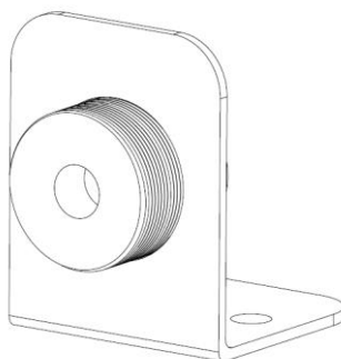
■ Abbildung 2-15 Gasanschluss-Module
