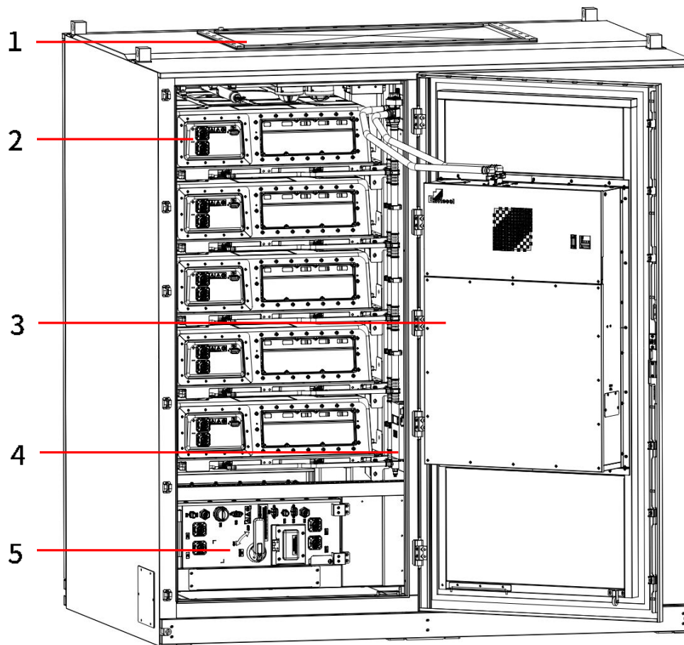
■ Abbildung 2-3 Batterieschrank – Innenraum -1
