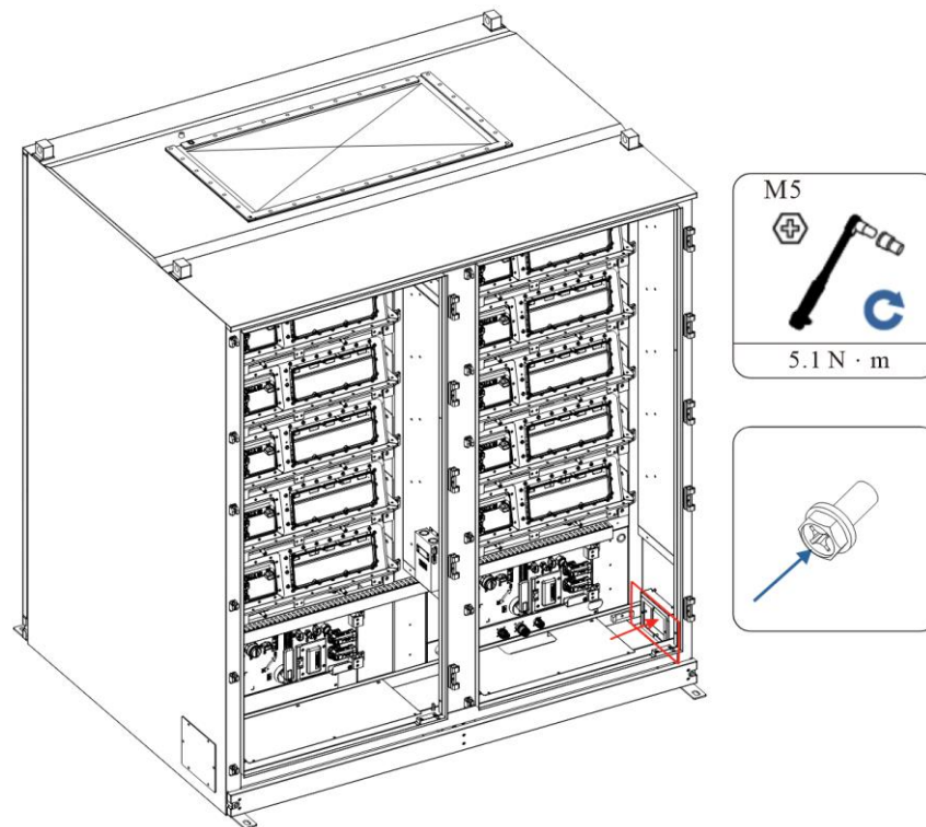
Abbildung 4-15 Installieren Sie die Spulendruckplatten
