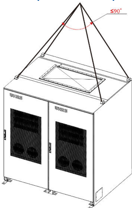
■ Abbildung 4-6 Verwenden Sie einen Kran, um den Schrank zur Installationsplattform zu bewegen
