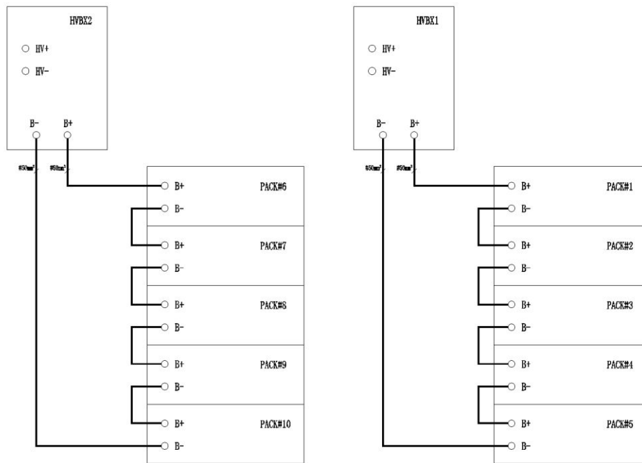
■ Abbildung 2-16 Schaltplan
