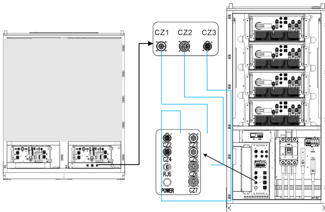
Abbildung 4-17 Installieren Sie die Kommunikationskabel
