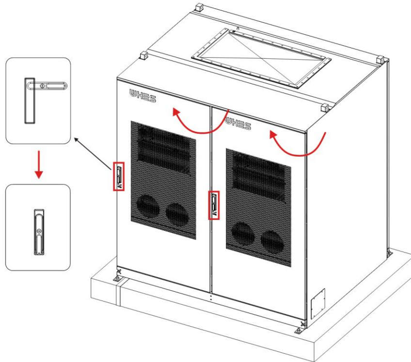
■ Abbildung 4-18 Schließen Sie die Vordertür des Schrankes
