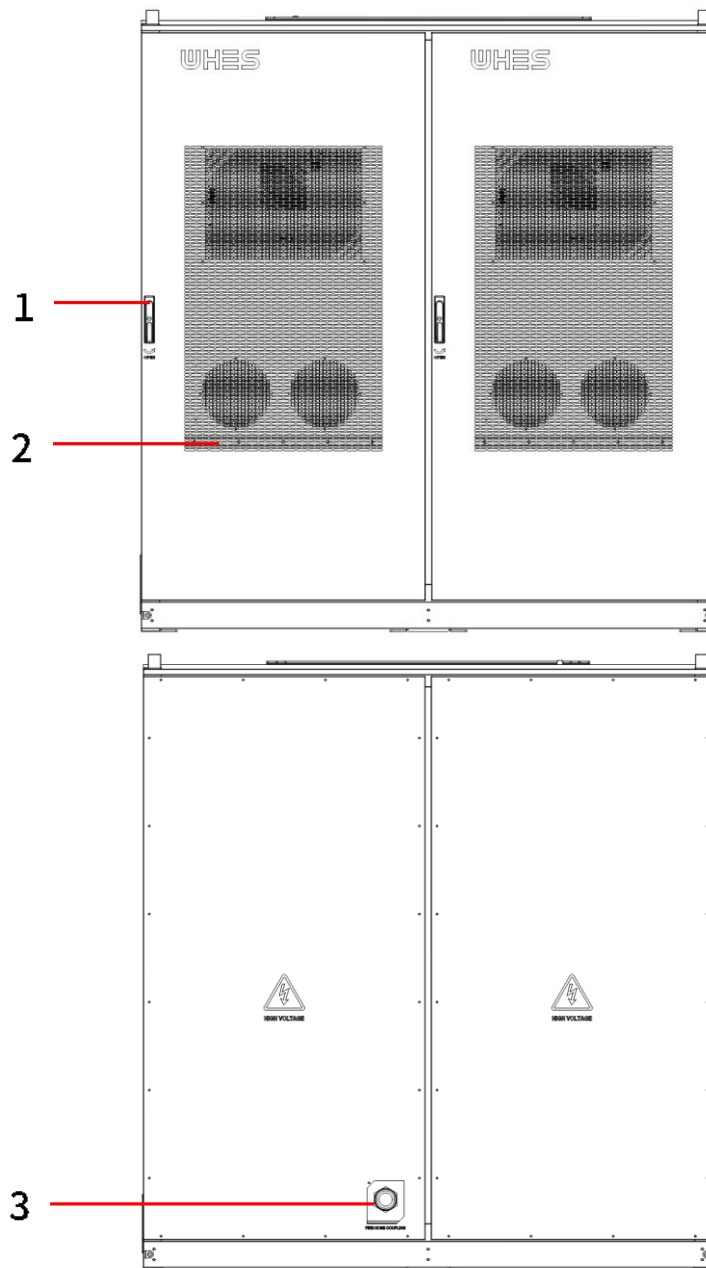
■ Abbildung 2-2 Batterieschrank – Vorder- und Rückansicht
