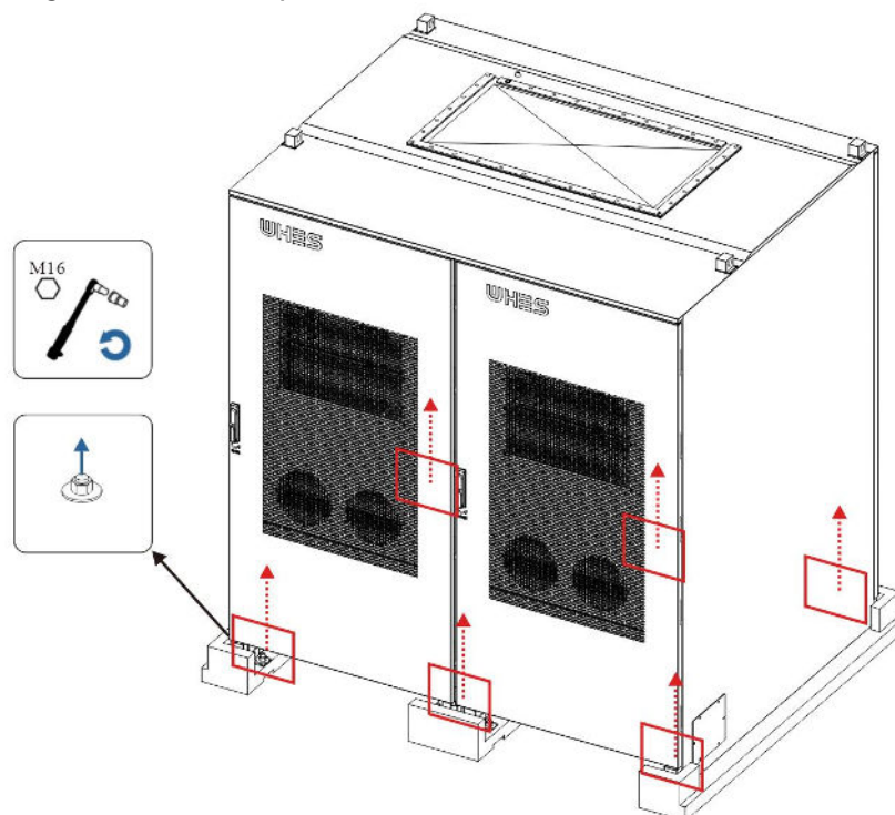
■ Abbildung 4-2 Zerlegen Sie die Holzpalette
