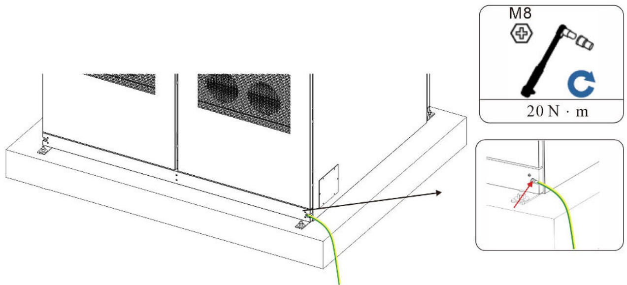
■ Abbildung 4-10 Installieren Sie den Erdungsdraht
