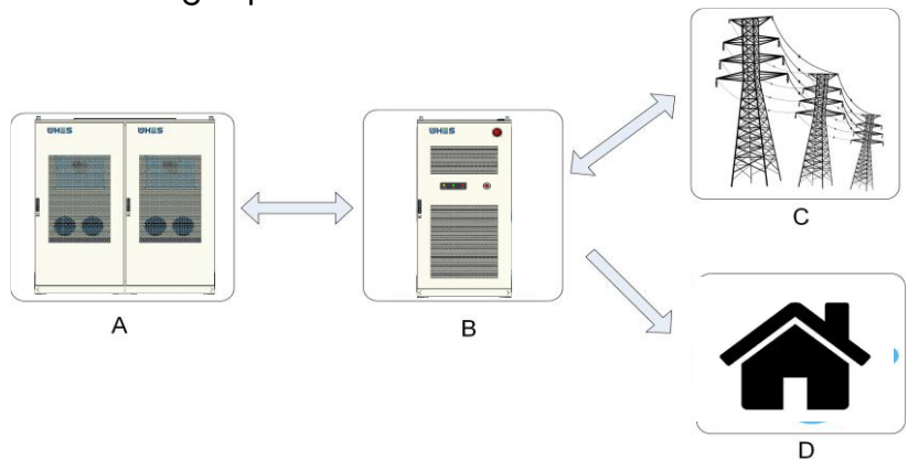
Abbildung 2-18 Anwendungsdiagramm für AC-Kopplungen
