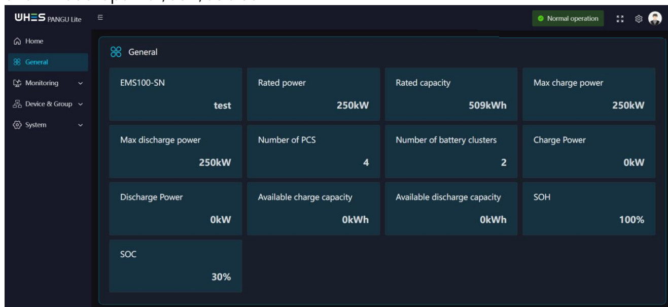
Abbildung 6-3 Übersicht über PANGU LITE
