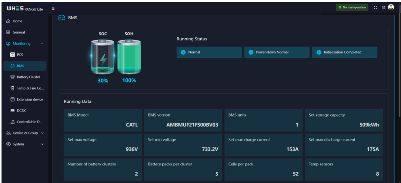
Abbildung 6-5 Betriebsüberwachung - BMS-Bildschirm
