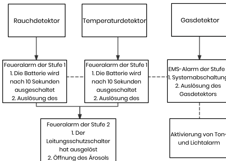
■ Abbildung 2-17 Feuerschutz-Logikdiagramm
