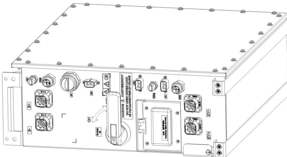
■ Abbildung 2-6 Aussehen des Hochspannungskastens
