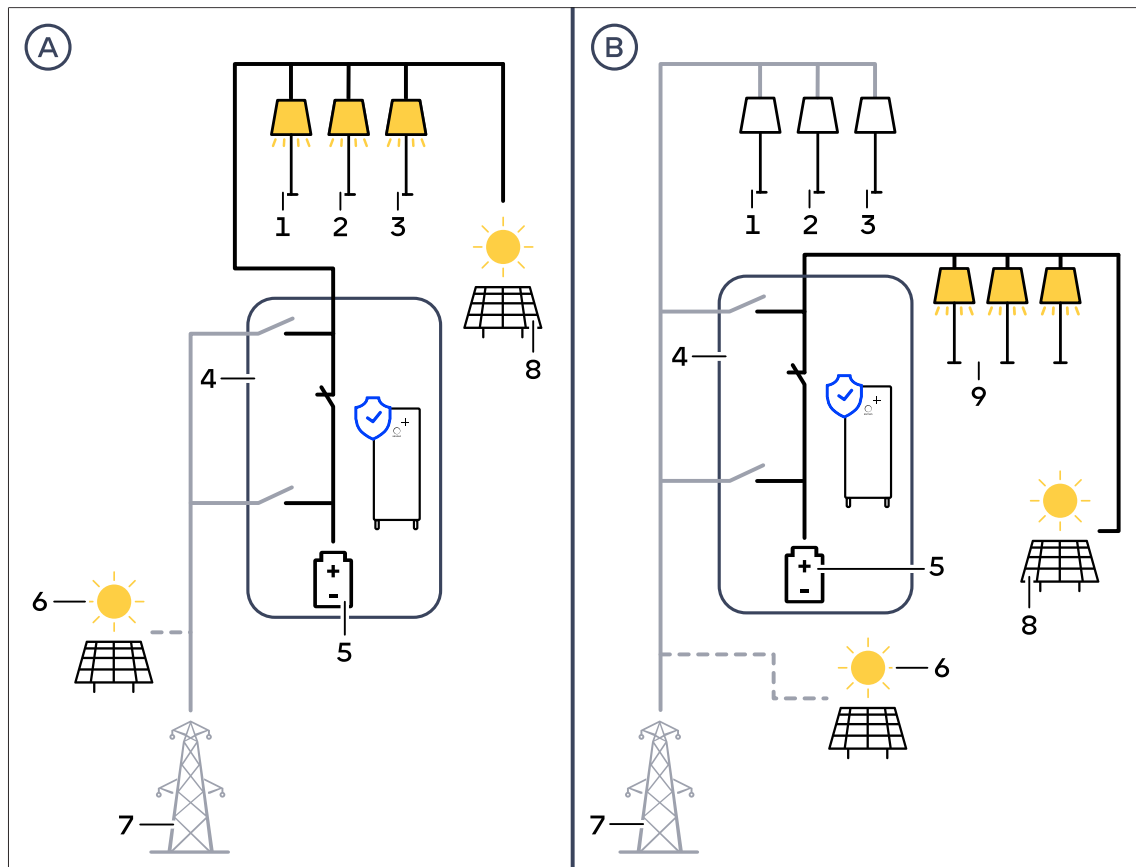
Abb. 9: Inselbetrieb - Netzausfall mit AC-Insel (A: Anschlussvariante 1; B: Anschlussvariante 2)
