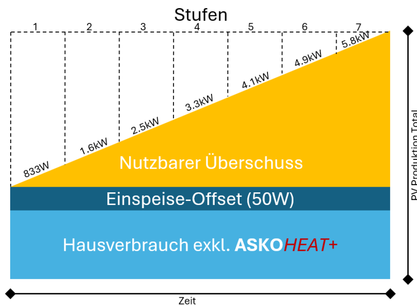
Beispiel eines 7-stufigen 5.8kW ASKOHEAT+ / + 2.0
