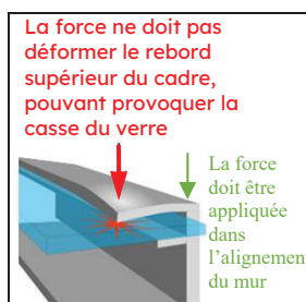
Figure 1a : Position de la Force de serrage de la bride
