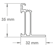
PROFIL DU PETIT CÔTÉ
