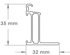
PROFIL DU GRAND CÔTÉ
