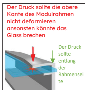
Abbildung 1a: Druck auf die Klemmenstellen
