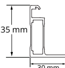
RAHMENPROFIL VON DER SEITE
